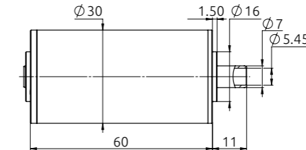
30 MM MOTOR
